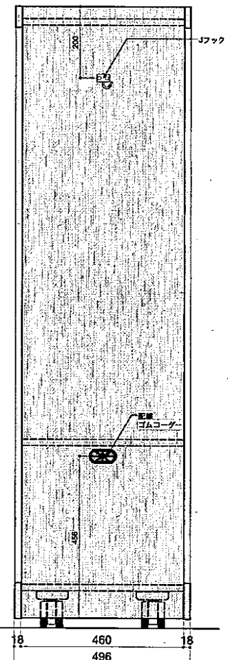
背面図 S=1:10
