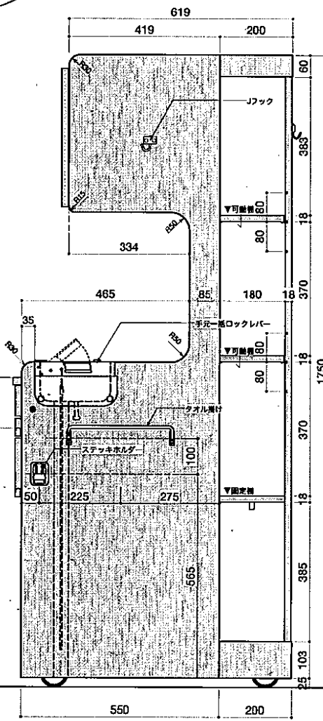
側面図B S=1:10
