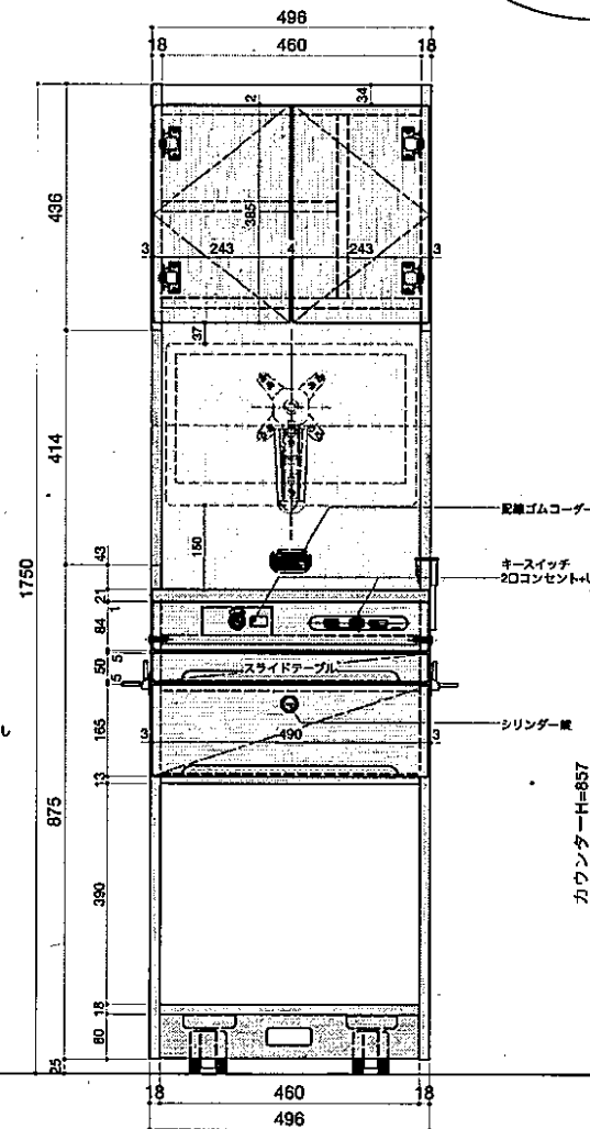
正面図 S=1:10
