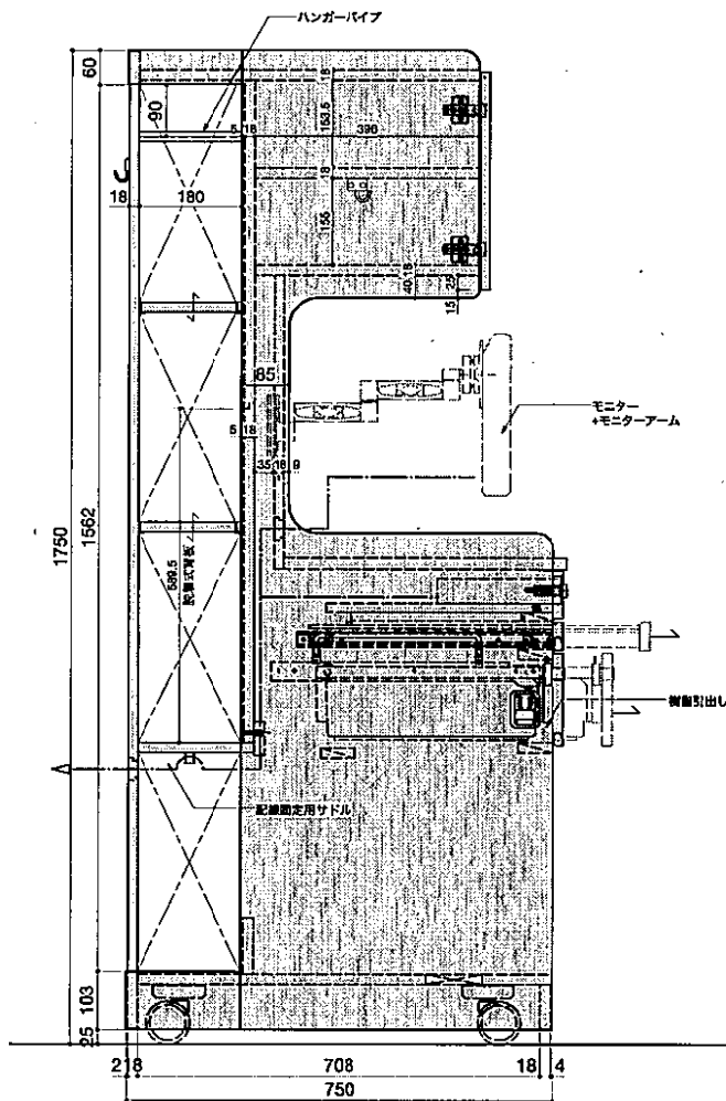
側面図A S=1:10
